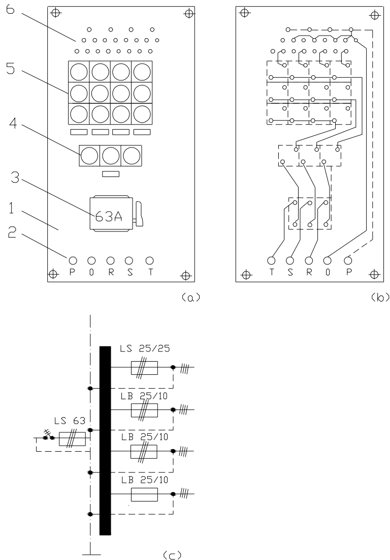
Fig. 10.1. Tablou de distribuție de marmură a - vedere din față; b - vedere din spate; c - schema monofilară.
